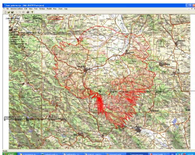
Sl. 4. Karta zone pokrivanja za hipotetički T-DAB predajnik sa lokacije MALJEN, portabilni prijem
